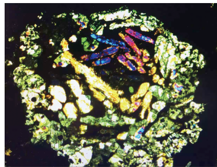
球粒陨石中“球粒”的正交偏光图像
